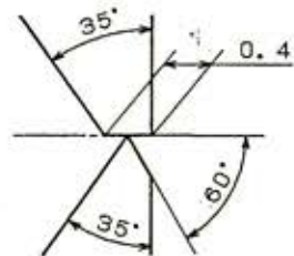
刃先拡大図 (10/1)
