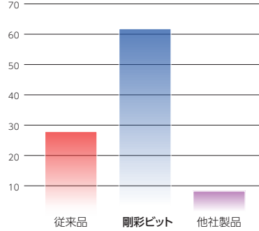
打ち込み試験 木材への打ち込み N=5 (本)
